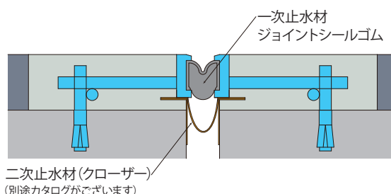
▲端部立ち上げ構造
