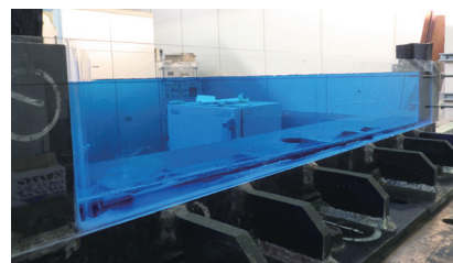
▲止水性能試験状況
