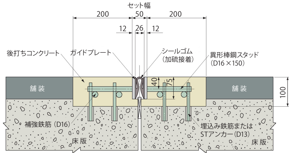
【断面図】
