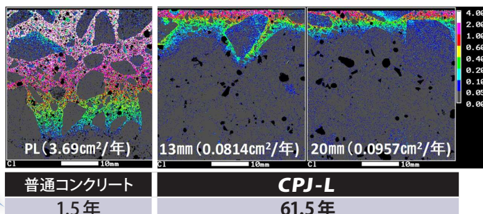
■ 塩化ナトリウム10%水溶液に、6ヶ月浸漬後のEPMAによる塩化物イオン拡散係数
