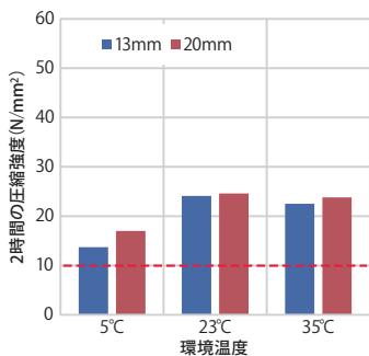
■ 2時間の圧縮強度
