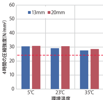
■ 4時間の圧縮強度
