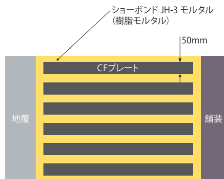
【平面配置図】
